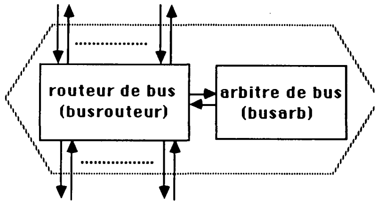
Fig. 17 Bus physique
